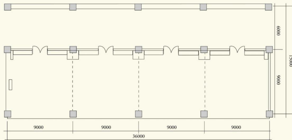
日月潭厅平面图
