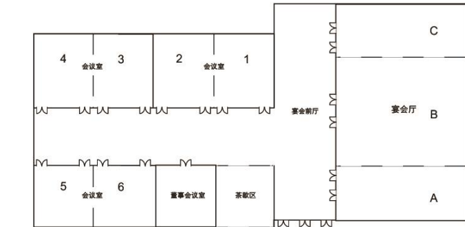
1层宴会厅及会议室平面图
