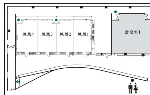
会议室区域平面图
