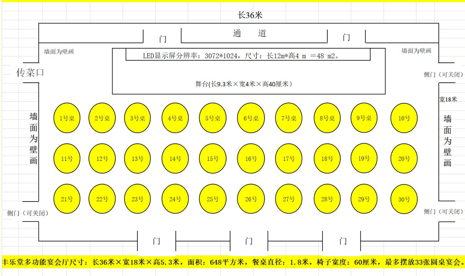
丰国祠食府一丰乐堂多功能宴会厅宴会平面图
